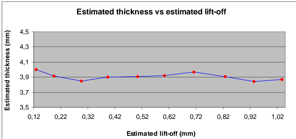
Figure 6. Epaisseur estimée sur lift-off estimé
