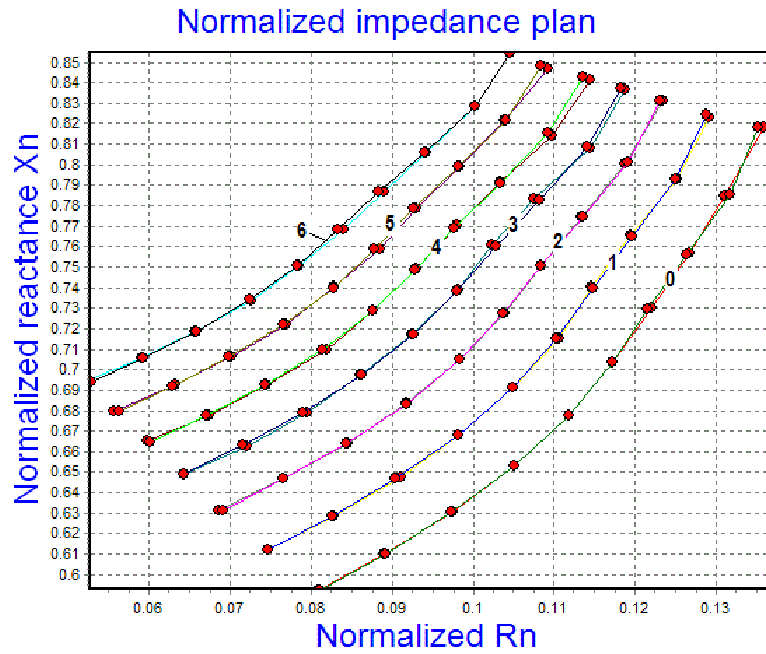
Figure 4. Courbes d'impédance normalisées multi-fréquences obtenues à 7 valeurs du lift-off. Le numéro de chaque courbe correspond au nombre de cales (0,1 mm d'épaisseur) insérées entre la sonde et la plaque
