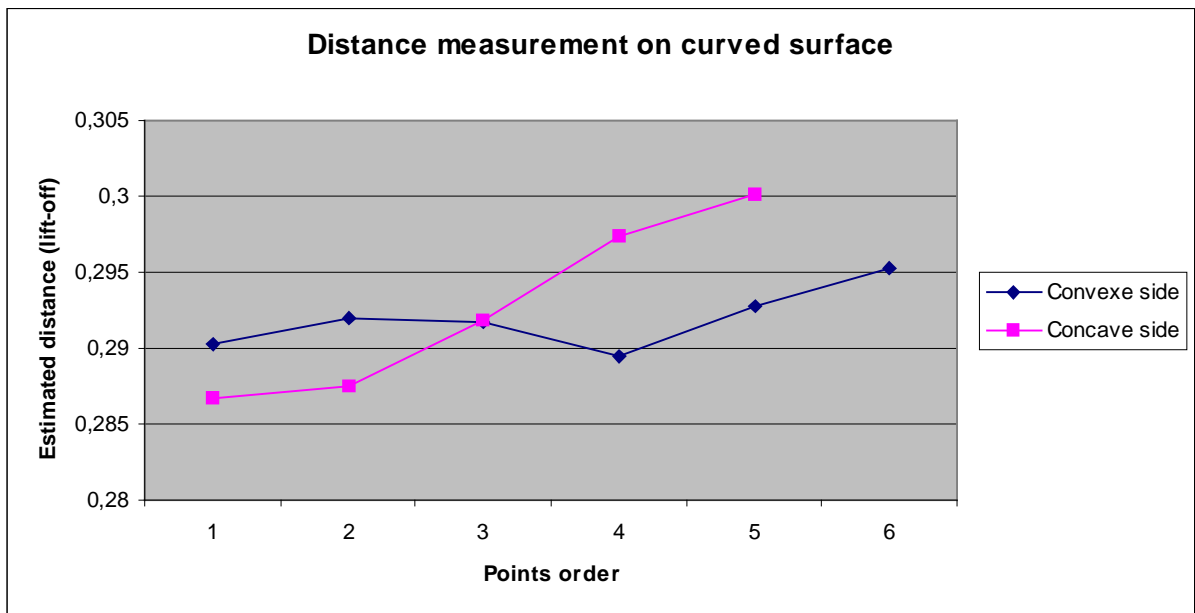
Figure 9. Valeurs du lift-off correspondant aux valeurs d'épaisseur estimée à la figure 8.
