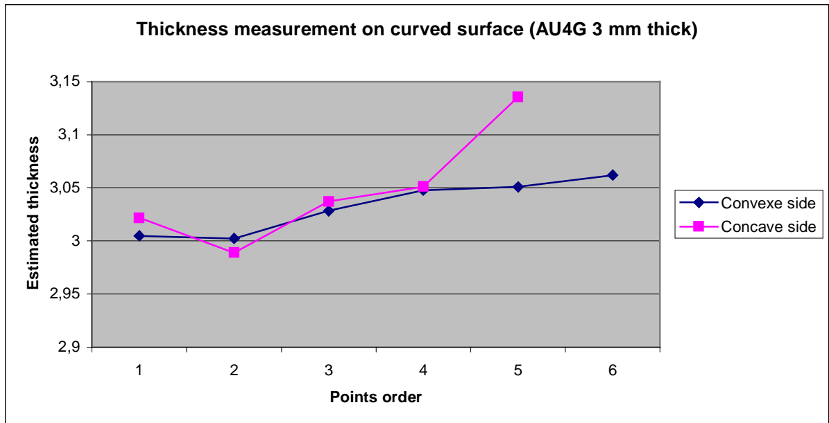
Figure 8. Résultat de mesure d'épaisseur sur les 2 faces de la plaque de coque d'avion
