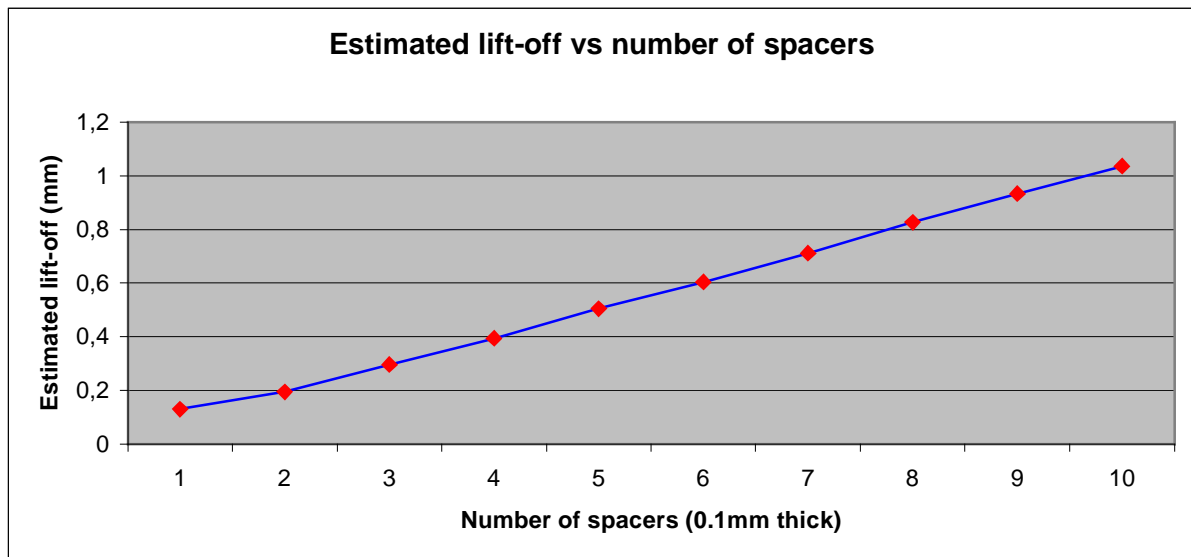
Figure 5. Estimation du lift-off par Conducens™ vs le nombre de cales de 0,1 mm d'épaisseur. Le résultat est quasiment linéaire.
