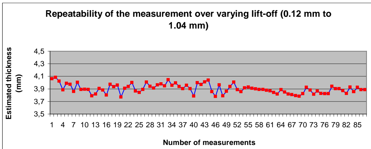
Figure 7. Répétabilité de la mesure de l'épaisseur sur 88 mesures, pendant que le lift-off varie de 0,12 mm à 1,04 mm. La valeur moyenne de l'épaisseur obtenue sur 88 mesures est de 3,903 mm.
