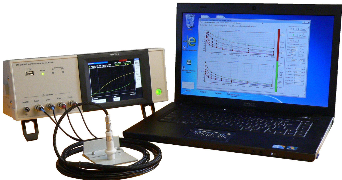
Figure 2. Conducens™ utilisant un analyseur d'impédance Hioki IM3570 qui va jusqu'à 5 MHz
